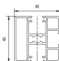
Kunststoff - Unterputztyp
