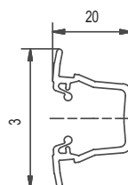
Kunststoff - Unterputztyp
