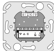
Thermis IB Tragrahmen Ansicht von hinten
